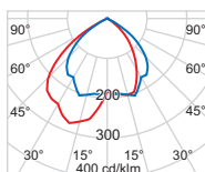
TC-DEL 2 x 26 W Halbstreuwinkel 53 / 30° Abschirmwinkel 34° Grenzausstrahlwinkel/1000 cd/m 2 65° Wirkungsgrad 55%
