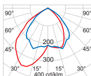
TC-DEL 2 x 18 W Halbstreuwinkel 50 / 30° Abschirmwinkel 34° Grenzausstrahlwinkel/1000 cd/m 2 65° Wirkungsgrad 64%
