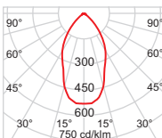
TC-TEL 26 W Halbstreuwinkel 2 x 29° Abschirmwinkel 46° Grenzausstrahlwinkel/1000 cd/m 2 60° Wirkungsgrad 59%
