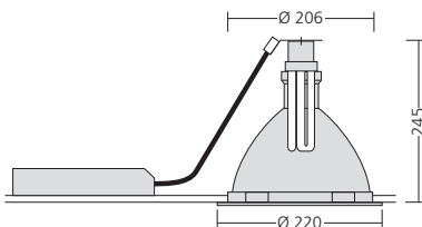
TC-TEL 26 W Halbstreuwinkel 2 x 29° Abschirmwinkel 46° Grenzausstrahlwinkel/1000 cd/m 2 60° Wirkungsgrad 59%
