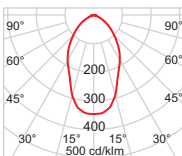
TC-TEL 42 W Halbstreuwinkel 2 x 32° Abschirmwinkel 34° Grenzausstrahlwinkel/1000 cd/m 2 80° Wirkungsgrad 53%
