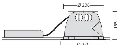
TC-DEL 2 x 18 W Halbstreuwinkel 50 / 30° Abschirmwinkel 34° Grenzausstrahlwinkel/1000 cd/m 2 65° Wirkungsgrad 64%
