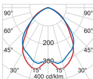
TC-DEL 2 x 26 W Halbstreuwinkel 2 x 45° Abschirmwinkel 14° Grenzausstrahlwinkel/1000 cd/m 2 75° Wirkungsgrad 78%
