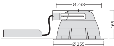
TC-DEL 2 x 26 W Halbstreuwinkel 2 x 41° Abschirmwinkel 43° Grenzausstrahlwinkel/1000 cd/m 2 55° Wirkungsgrad 57%
