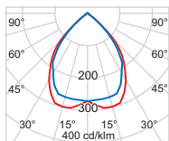
TC-TEL 2 x 32 W Halbstreuwinkel 2 x 42° Abschirmwinkel 43° Grenzausstrahlwinkel/1000 cd/m 2 55° Wirkungsgrad 49%
