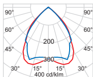
TC-DEL 2 x 26 W Halbstreuwinkel 2 x 41° Abschirmwinkel 43° Grenzausstrahlwinkel/1000 cd/m 2 55° Wirkungsgrad 57%
