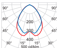
TC-DEL 2 x 18 W Halbstreuwinkel 2 x 42° Abschirmwinkel 14° Grenzausstrahlwinkel/1000 cd/m 2 70° Wirkungsgrad 73%
